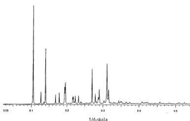
Figur 1. Røntgenstrålepulverdiffraktionsgram af omeprazol form A målt med variable spalter
