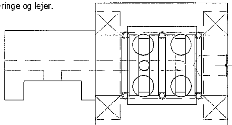
Figur 1 – Komplet vakuumsvirvel
