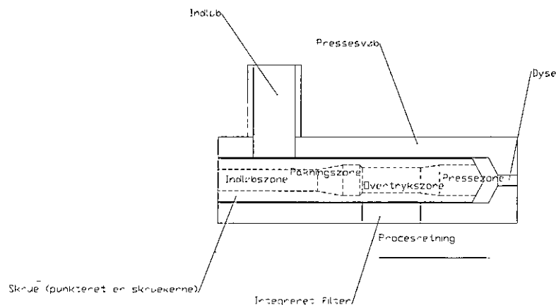
Figur 1: Principskitse af opbygning af pressen, og udformning af skruen
