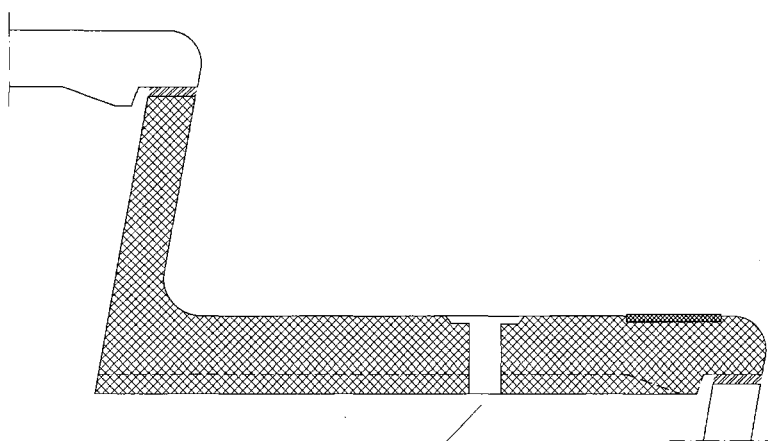
Eksempel på udsparring for ankerbolt.
