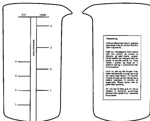
Figur 5 Et eksempel på en foretrukket udførelsesform "Den cylinderveformede og koniske portionsmåler"
